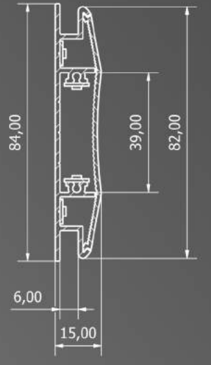
A-A ( 1 : 1 )
